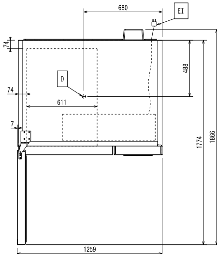
Felülnézet
